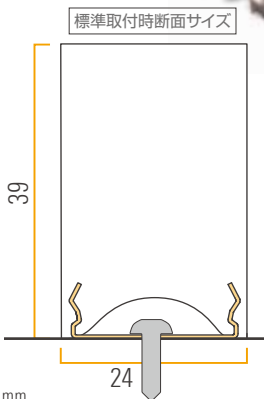
標準取付時断面サイズ
