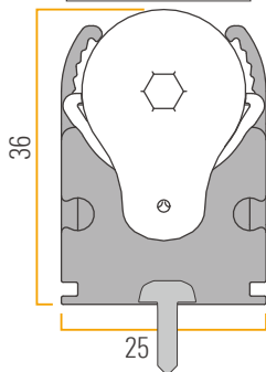
標準取付時断面サイズ
