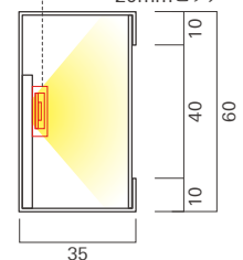
A-A' 断面図
