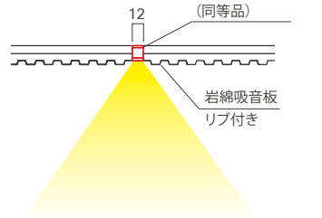
Detail A 断面図
