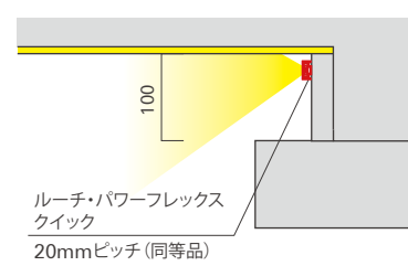
Detail B 断面図
